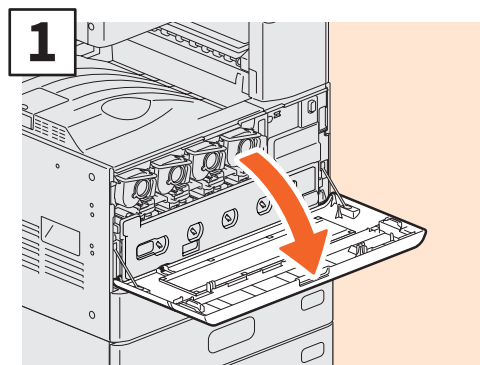
1 Öppna frontluckan.
