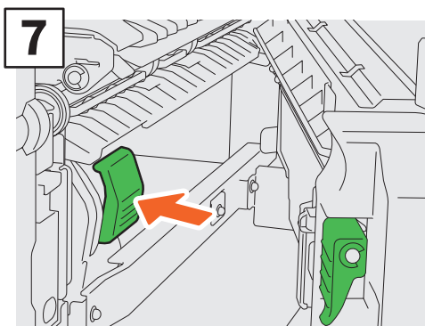
7 Installera klammerkassetten.
