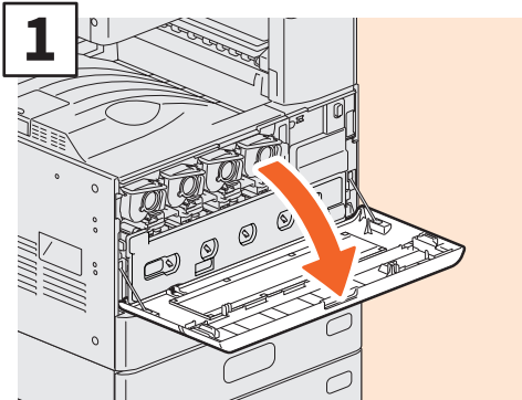
1 Öppna frontluckan.
